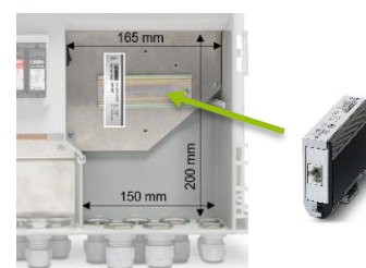
DINレールによる拡張可能 (RJ45避雷器等)
