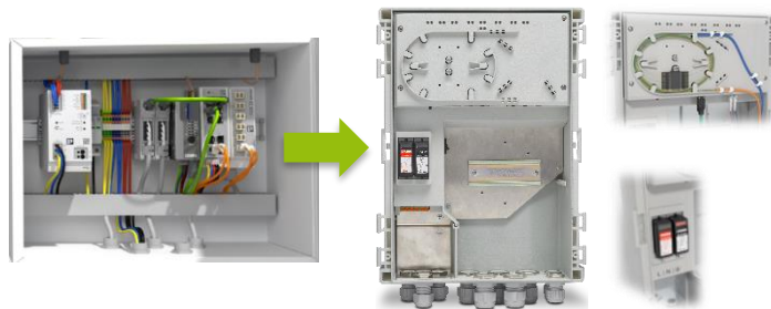
盤内機器の電源系統配線が不要で、光配線もキレイに収納 一次側の過電圧保護機能を標準装備
